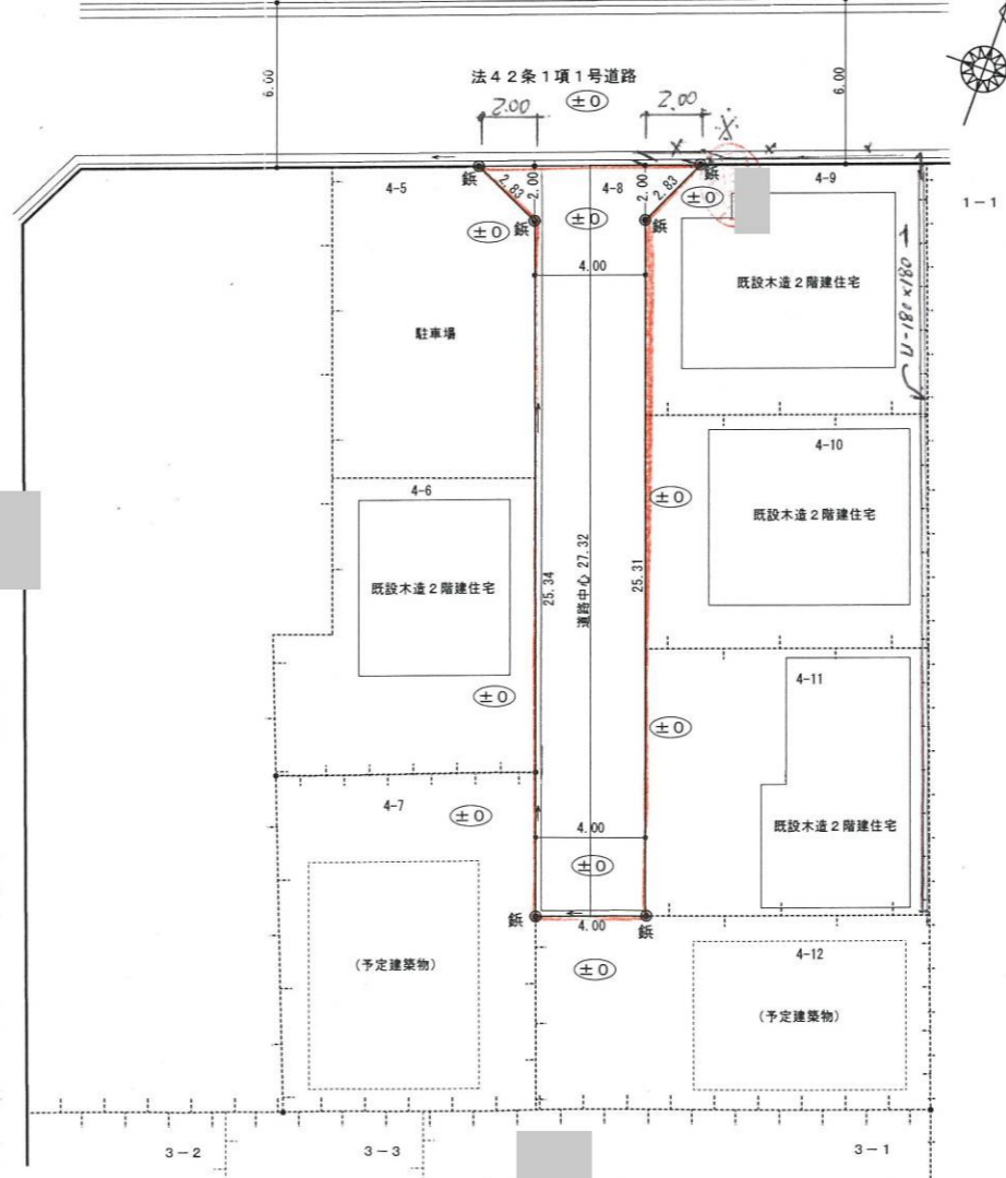
道路図(平面図) S:1/300
