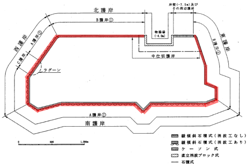
図 2-3-3 護岸等の構造及び配置図
