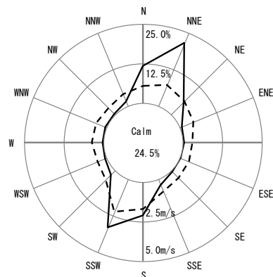
図 10.13-6 W-2 における風配図
