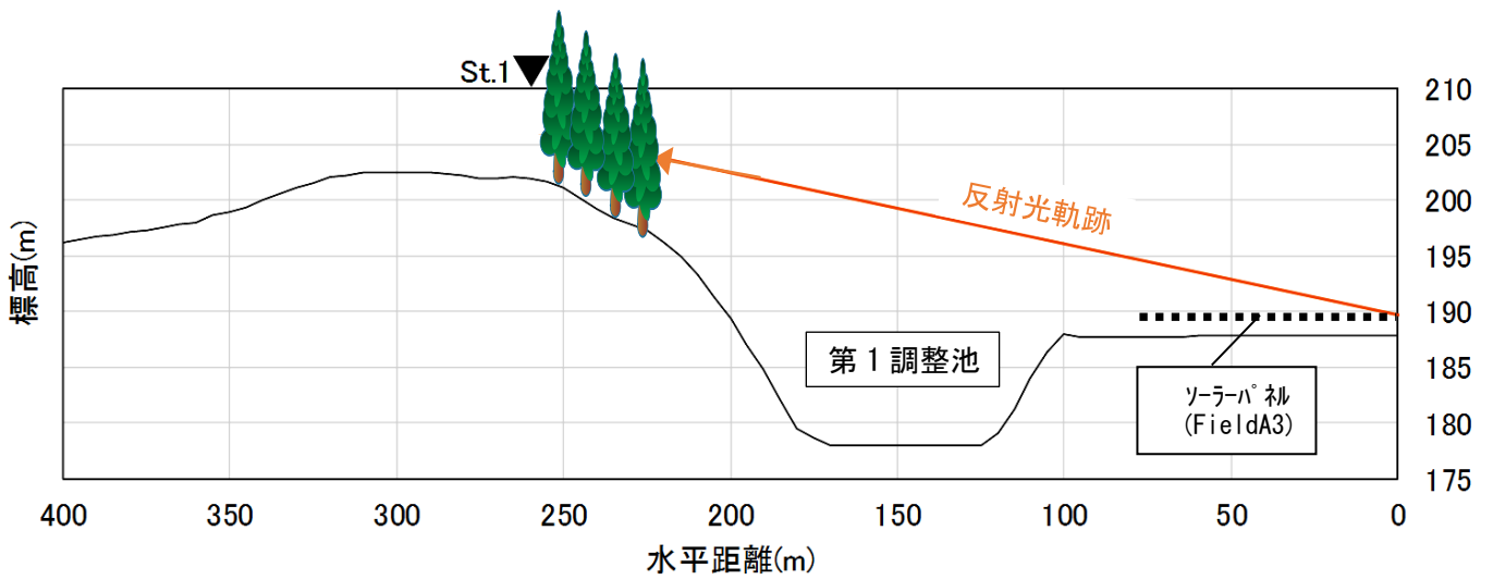
図 10.12-5 (2) 樹林の遮蔽効果を考慮した場合の夏至における予測結果（St.1）
