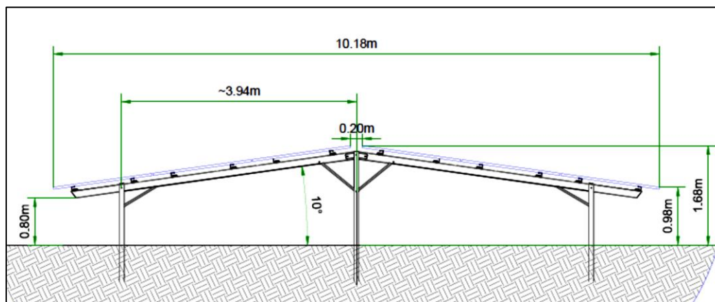
図 10.12-1 パネルの配置図（Field A1～A3, B, G）
