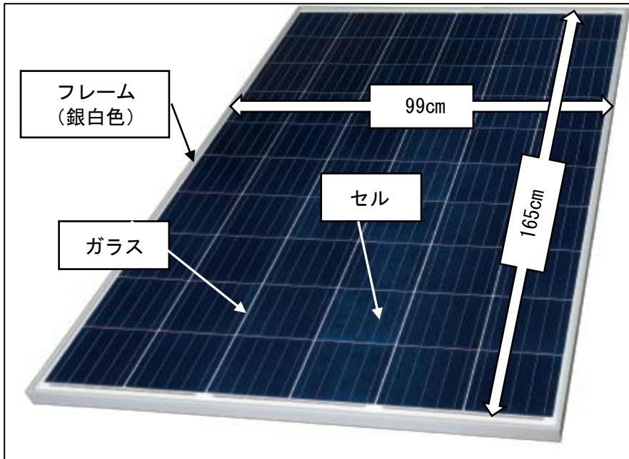
図 10.12-7 ソーラーパネルの仕様
