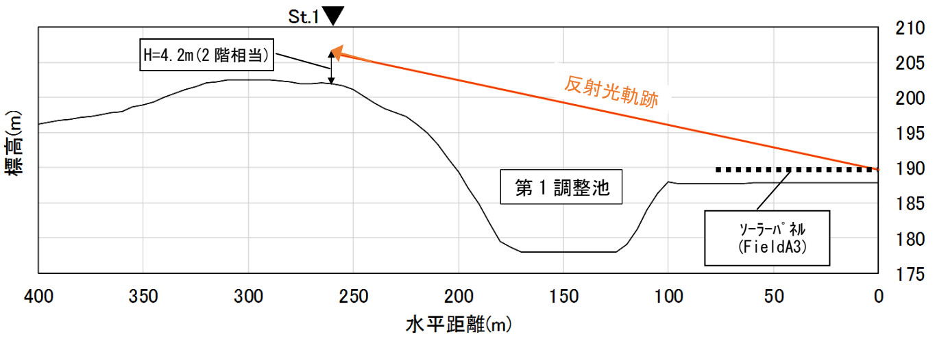
図 10.12-3 (2) 夏至における予測結果 (St.1)
