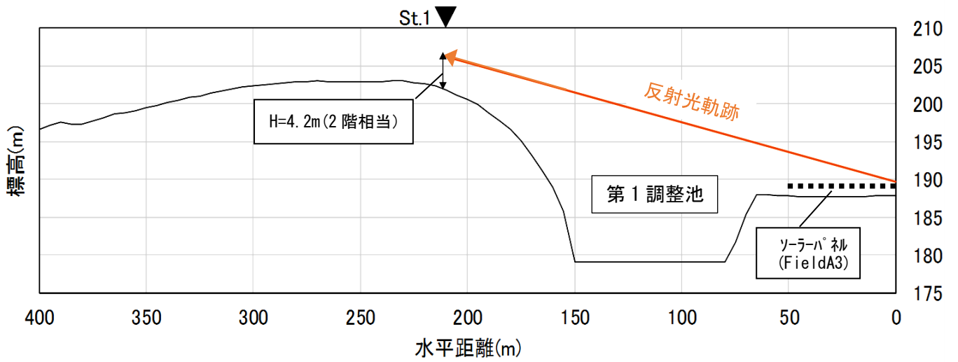
図 10.12-3 (1) 春分 (秋分) における予測結果 (St.1)
