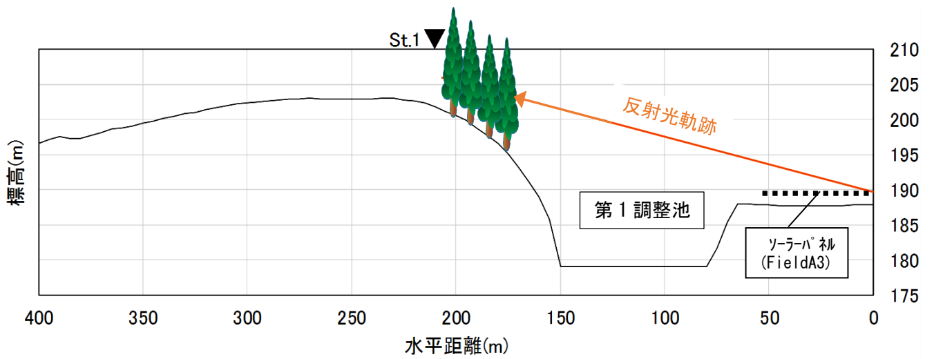
図 10.12-5 (1) 樹林の遮蔽効果を考慮した場合の春分（秋分）における予測結果（St.1）
