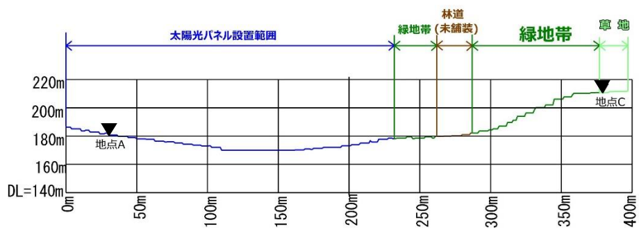
図 10.13-2 調査地点の概念図と横断図
