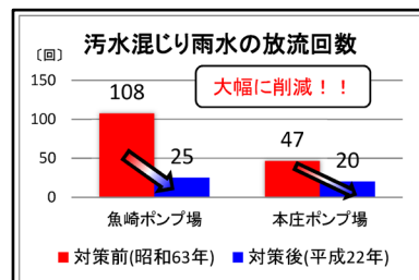
合流式下水道改善事業（貯留施設の整備）と事業効果
