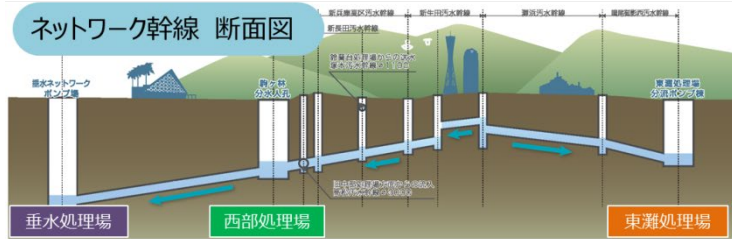
処理場間ネットワークシステムの仕組み
