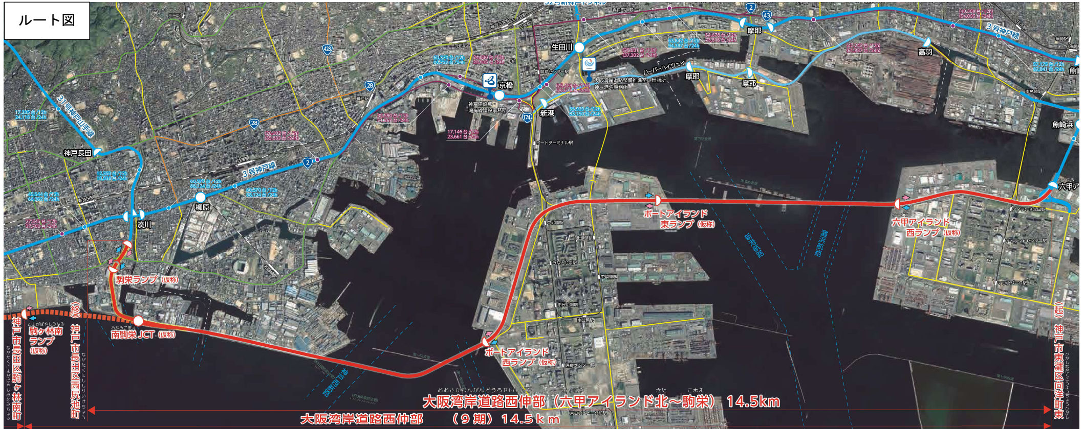
縦断図 (※構造については、現時点の計画であり、今後変更される可能性があります。)
